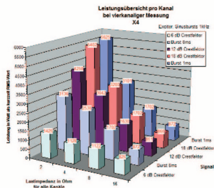
Leistungswerte bei gleichzeitiger Belastung aller Kanäle mit Sinusburst und Burstsignalen mit verschiedenen Crestfaktoren. (Leistungsangaben als Kurzzeit RMS-Werte aus V_{peak} berechnet) (Abb. 21)
