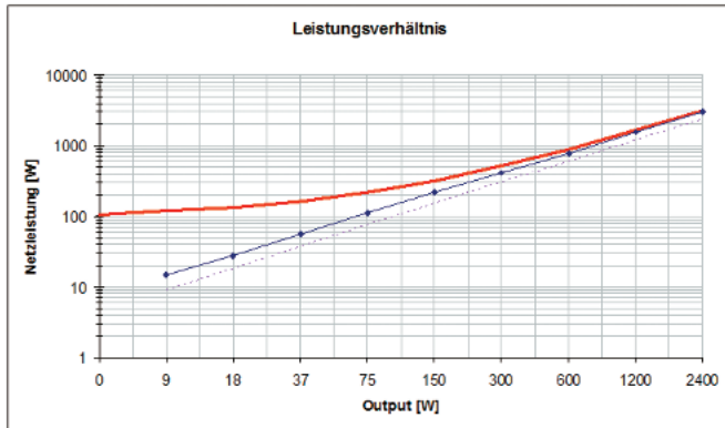
Leistungsverhältnis Abgegebene Leistung (x-Achse) in Relation zur aufgenommenen (y-Achse) als rote Kurve. In blau die Werte abzüglich der Grundlast von W, die die Endstufe erzeugt. In rosa die Idealkurve für 100 % Wirkungsgrad (Abb. 22)
