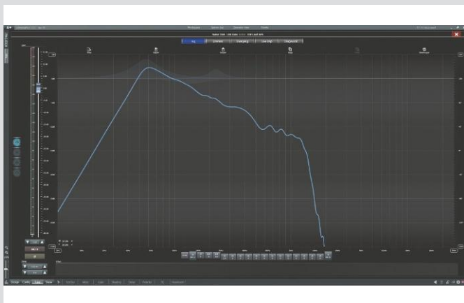
FIR-Filter im CSV-Format importiert die Armonía-Software mit 48 kHz Abtastrate und einer Länge bis zu 2048 Taps. Die Grafik zeigt das FIR-Filter für den Tieftöner zusammen mit einem Hochpass und drei Bell-Filtern, die als IIR-Filter umgesetzt werden (Abb. 20)
