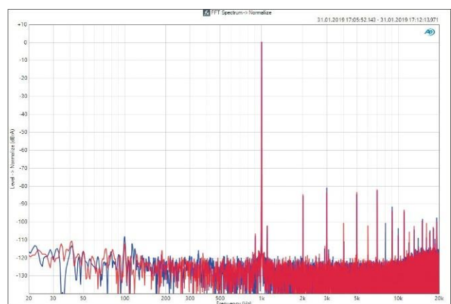
Klirrspektrum (THD+N) der T602 bei 1 kHz (CH1, CH2) mit einer Leistung von 2 × 500 W an einer 4-Ω-Last (Abb. 10)
