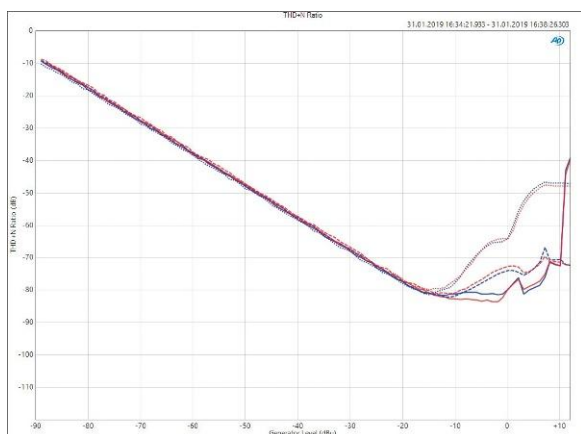
Klirrfaktor (THD) der T602 bei 100 Hz (durchgezogen), 1 kHz (gestrichelt) und 6,3 kHz (gepunktet) (CH1, CH2) in Abhängigkeit vom Eingangspegel auf der x-Achse an 4-Ω-Last (Abb. 9)
