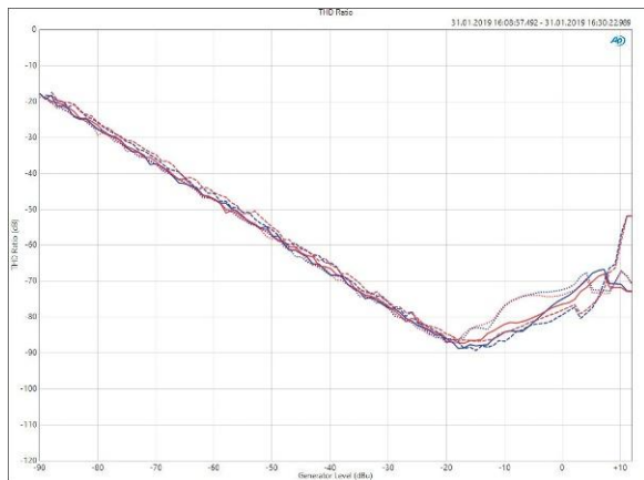
Klirrfaktor (THD) der T602 bei 1 kHz (CH1 rot, CH2 blau) in Abhängigkeit vom Eingangspegel auf der x-Achse an 2 Ω (gepunktet), 4 Ω (durchgezogen) und 8 Ω (gestrichelt) Last (Abb. 7)
