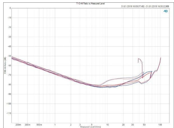
Klirrfaktor (THD) der 4804 bei 1 kHz (CH1 rot, CH2 blau) in Abhängigkeit von der Ausgangsspannung auf der x-Achse mit Belastungen von 2 Ω (gepunktet), 4 Ω (durchgezogen) und 8 Ω (gestrichelt). Beim Einsatz der Limiter bricht die Kurve ab oder wird rückläufig (Abb. 8)
